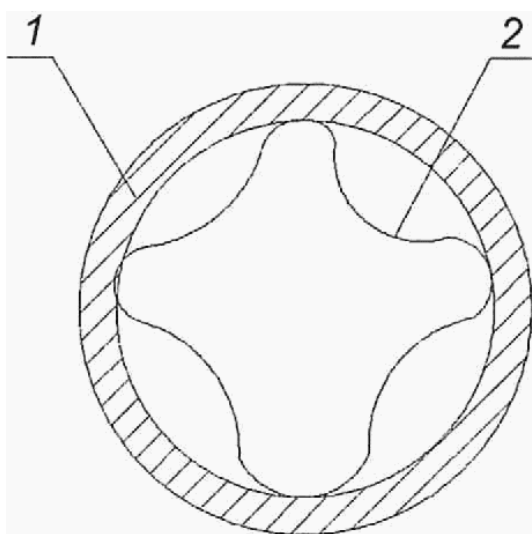
1 - муфта; 2 - уплотнитель
